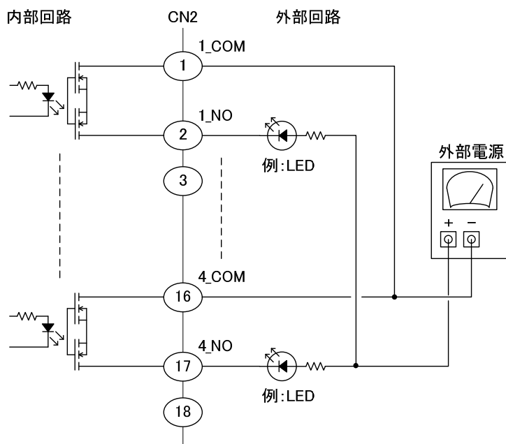
出力部接続例
