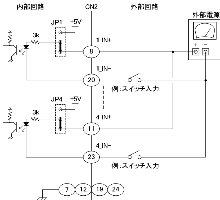
入力部接続例(外部電源使用)
